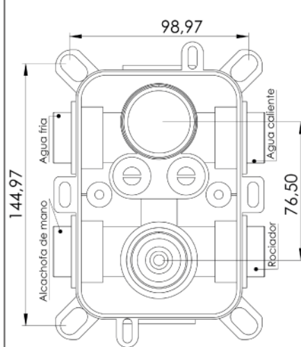
CROKIS CUERPO DE GRIFERIA CROKIS FAUCET BODY
